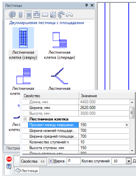
Рисунок 23.4.8. Образец выполнения самостоятельной работы 1.4..
